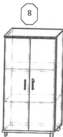
Skriňa 2 dverová Výška 1140 mm Šírka 600 mm Hĺbka 350 mm
