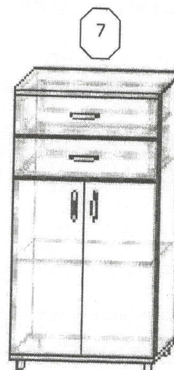
Skriň.2dv.+2zásuv. Výška 1140 mm Šírka 600 mm Hĺbka 350 mm
