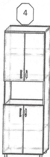
Skriňa 4 dverová Výška 1850 mm Šírka 600 mm Hĺbka 350mm
